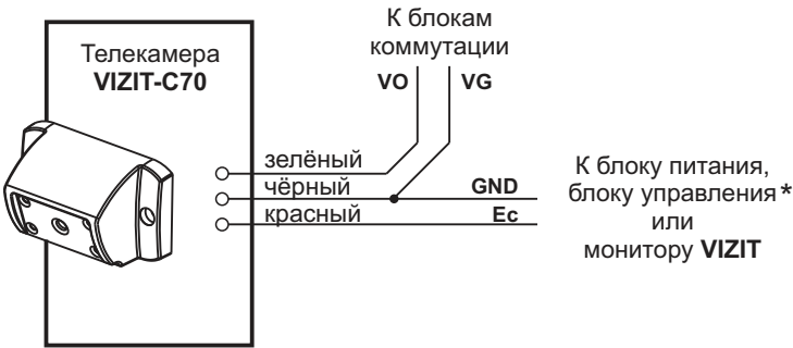
Рисунок 5 - Подключение VIZIT-C70
