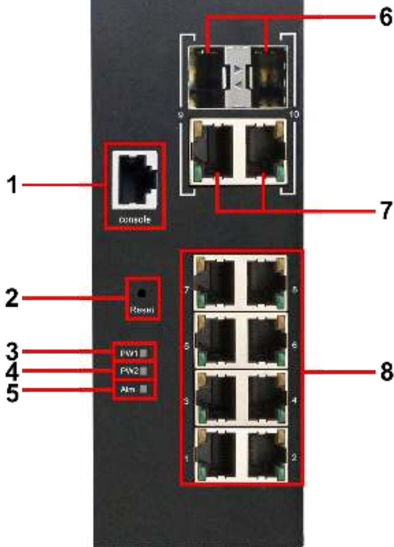
Рис. 2 Коммутаторы SW-60822/ILC (SW-80822/ILC), разъемы, кнопки и индикаторы передней панели
