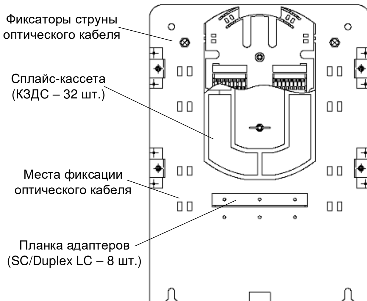
Рисунок 3.4 - Оптический кросс
