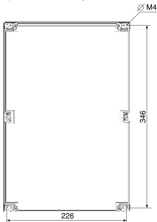
Рисунок 7.1 - Разметка крепления
