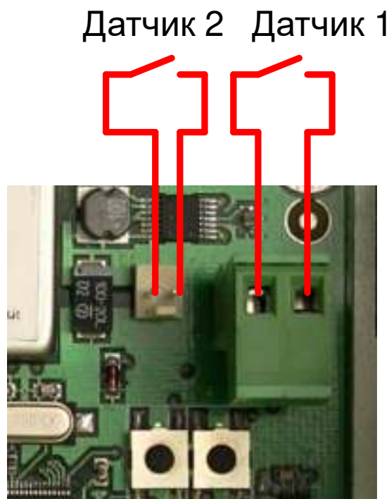
Рисунок 3.6 - Сухие контакты
