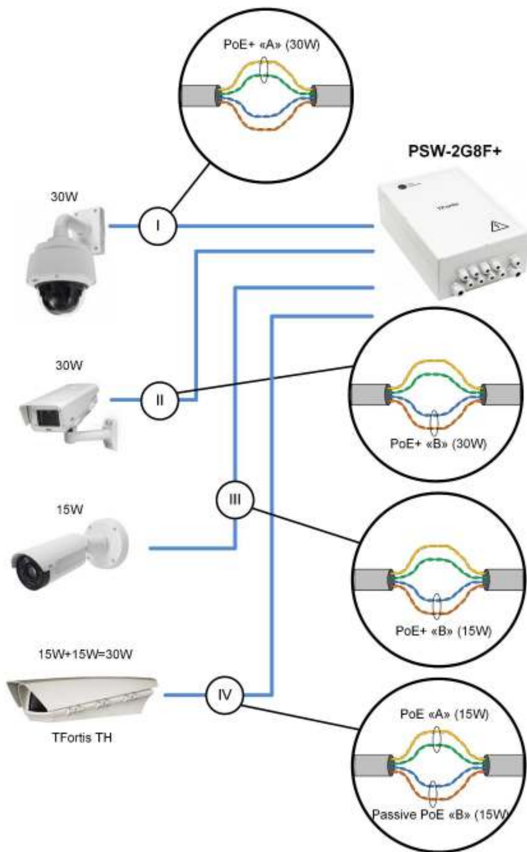
Рисунок 3.3 - Схема питания по PoE для разных случаев
