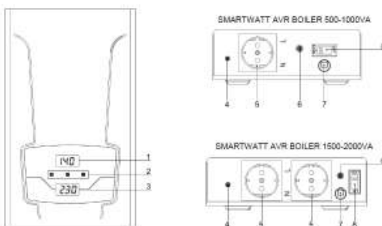
Рисунок 1. Внешний вид стабилизаторов напряжения SMARTWATT AVR BOILER 500-2000VA. Описание элементов приводится в таблице 1.
