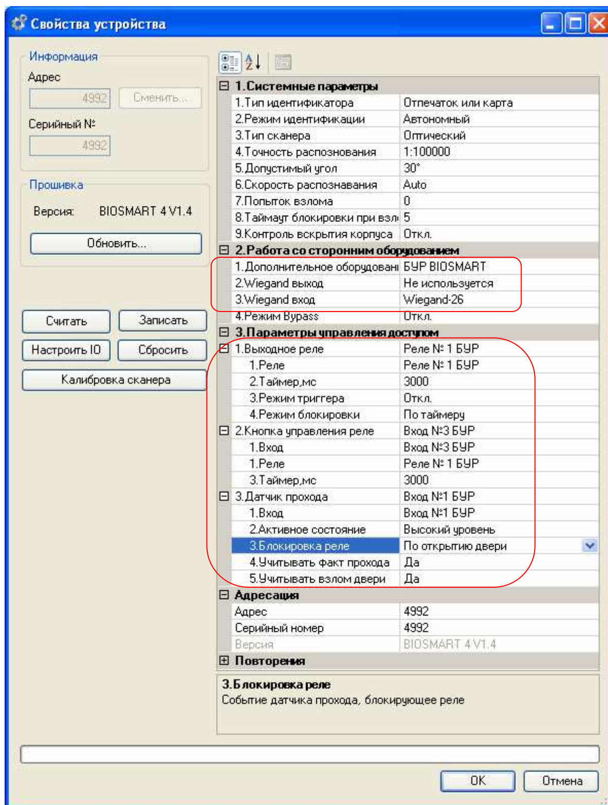
Рисунок 6 - Значение параметров контроллера №1.
