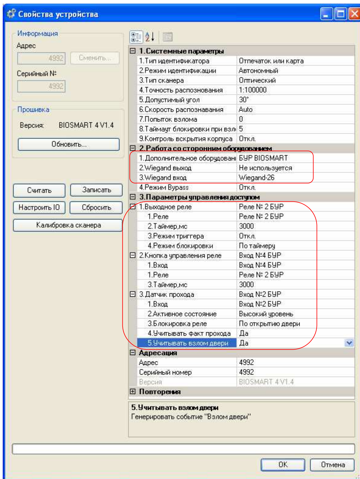
Рисунок 7 - Значение параметров контроллера №2.
