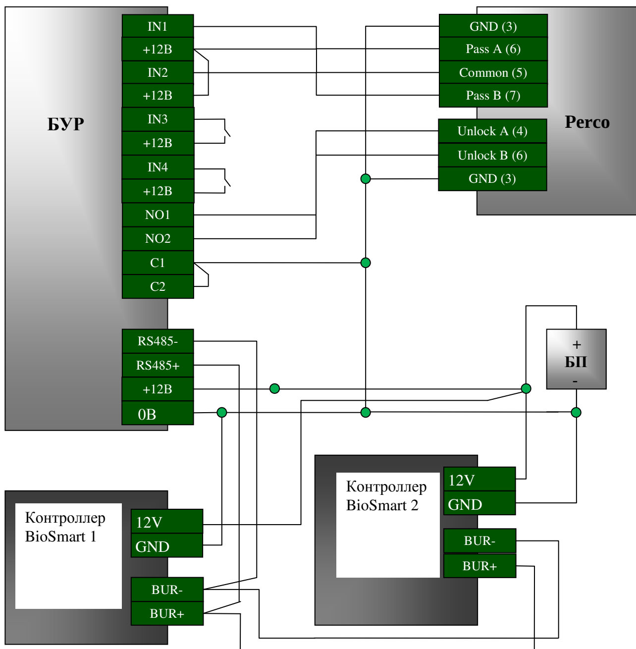
Рисунок 5 - Подключение контроллеров и БУР к турникету.
