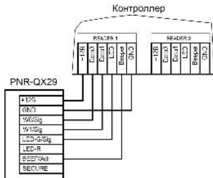
Рисунок 7. Подключение считывателя по интерфейсу Wiegand
