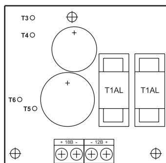
Рисунок 1 - Расположение элементов на плате блока питания БПД18/12-1-1
