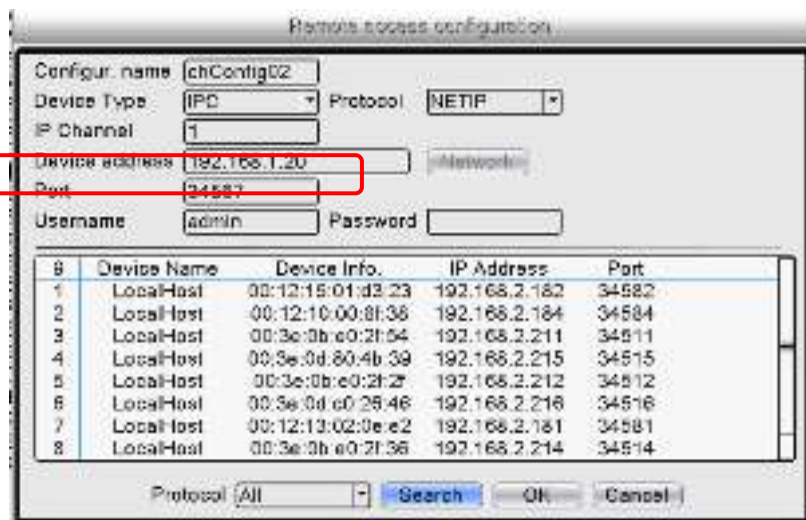
Рис.4.15 Поиск камер
