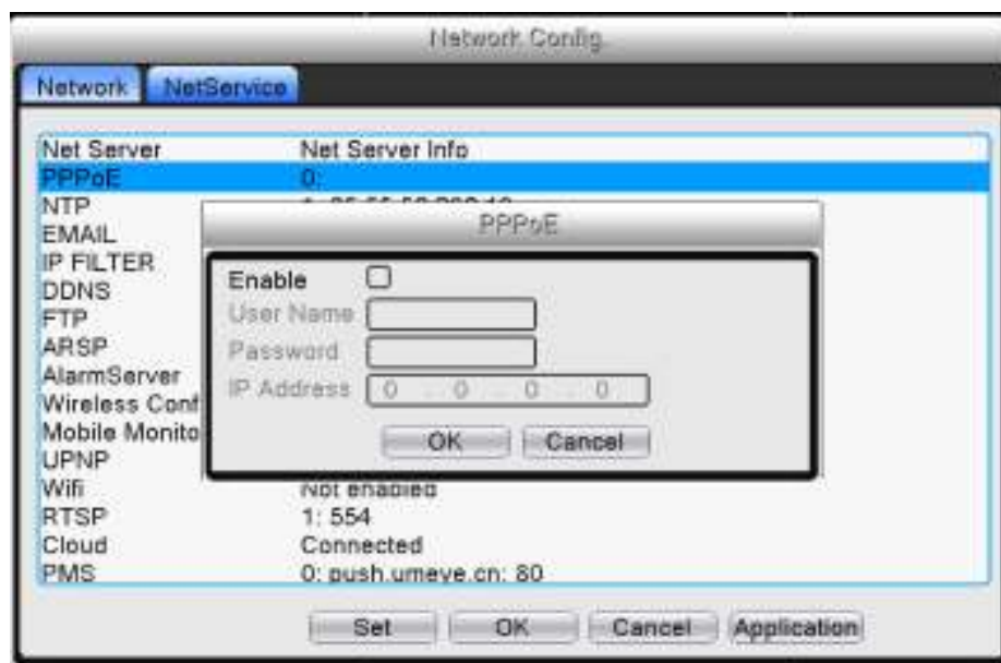
Рис.4.25 Настройки PPPOE
