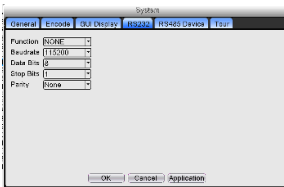
Рис.4.43 RS232
