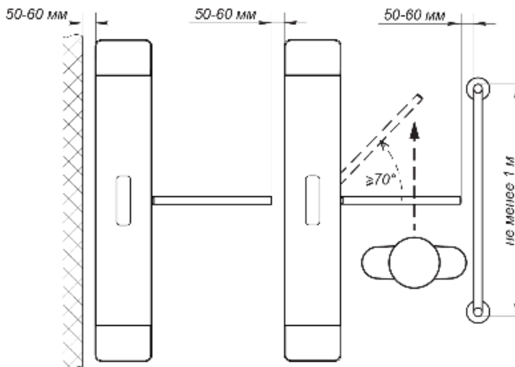
Рисунок 14. Рекомендации по организации зоны прохода
