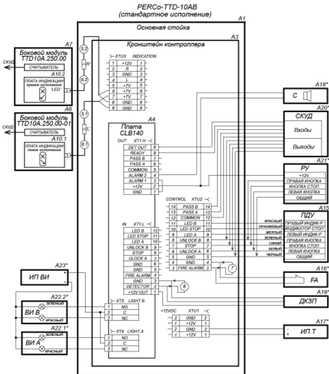
Рисунок 17. Схема соединений турникета и дополнительного оборудования для стандартной модификации PERCo-TTD-10AB 1
