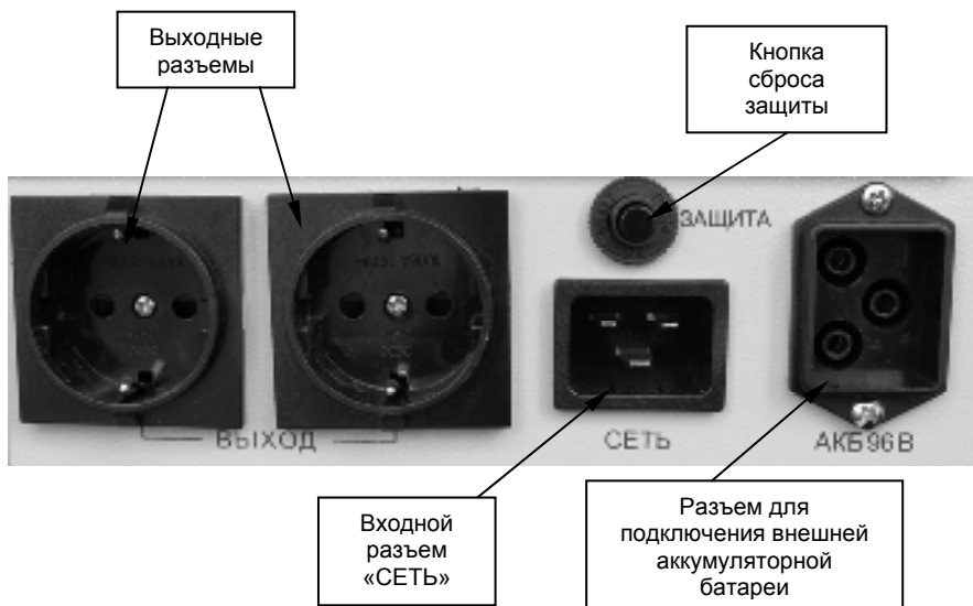
Рисунок 1 – Задняя панель источника
