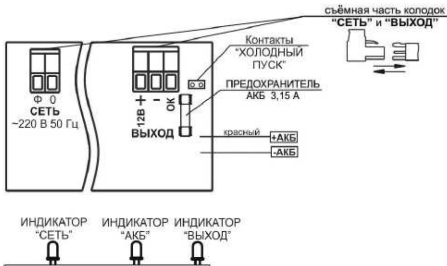
Рисунок 2 - вид изделия с открытой крышкой
