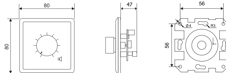
Габариты и установочные размеры (мм)
