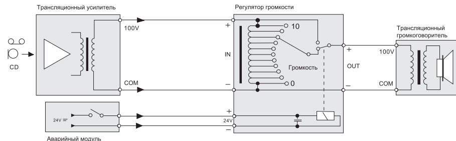
Схема подключения
