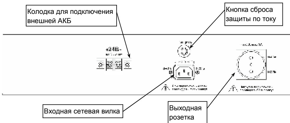
Рисунок 2 — Общий вид задней панели изделия.
