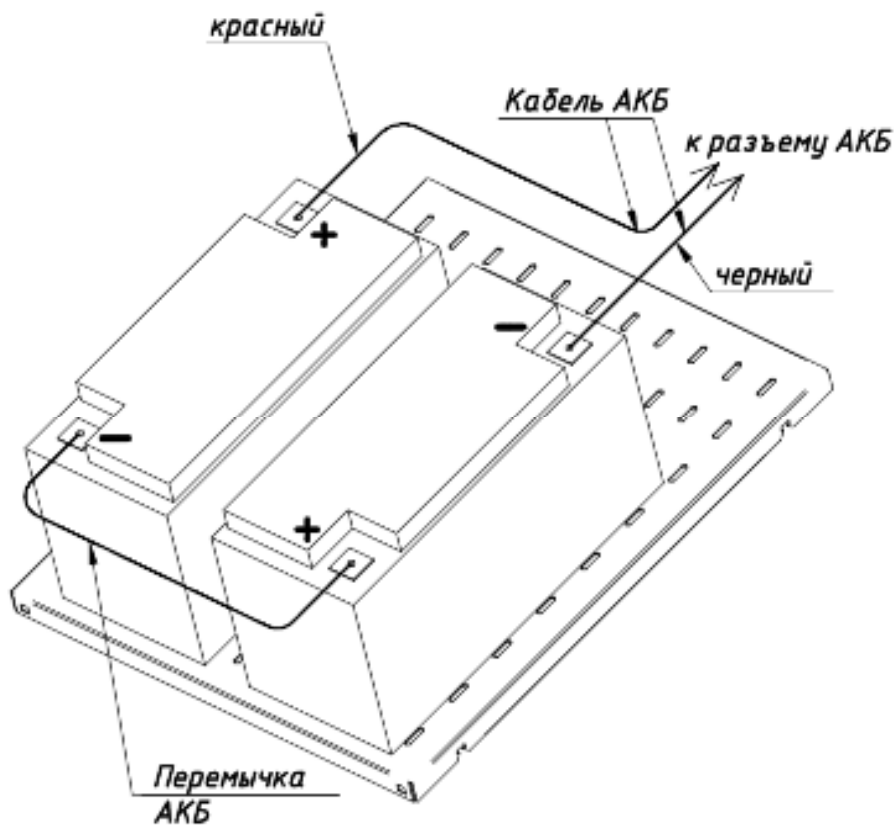
Рисунок 3 — Схема подключения аккумуляторных батарей
