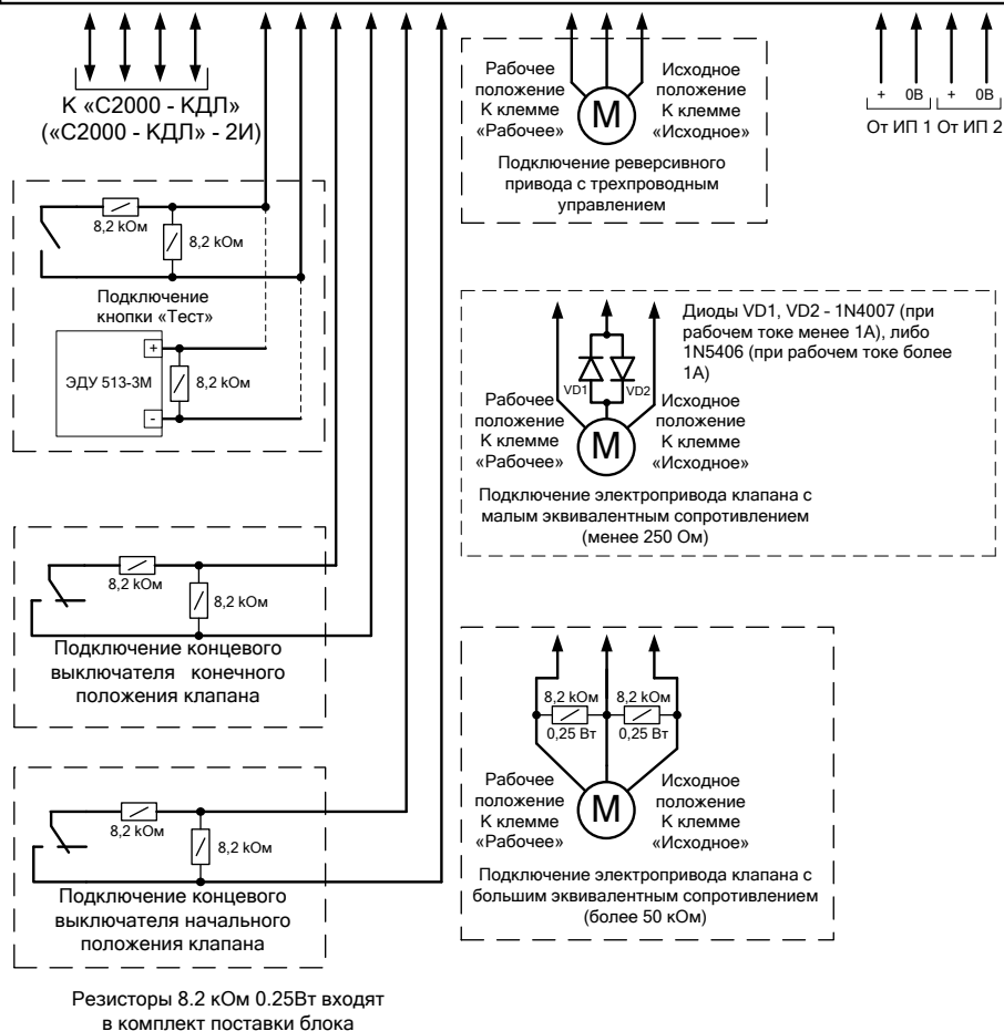
Рисунок 4. Схема внешних соединений блока
