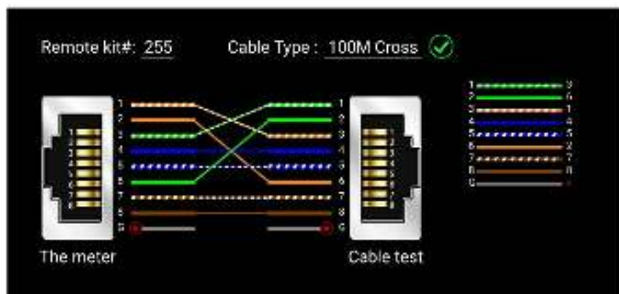
Рис.17 Тест «кроссового» кабеля
