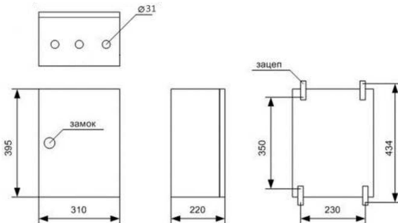
Рисунок 4 – Чертеж
