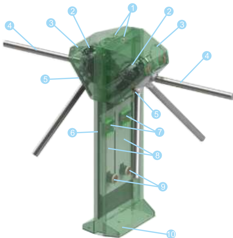
Рисунок 6.1 Внешний вид турникета «STL-04»
