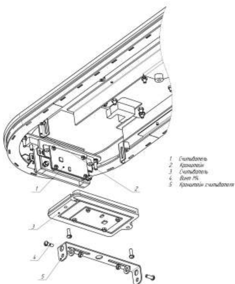
Рисунок 13 – Схема установки считывателя бесконтактных карт
