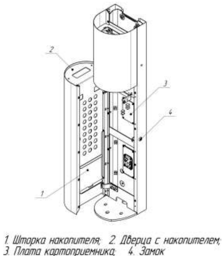
Рисунок 10 – Общий вид стойки картоприемника
