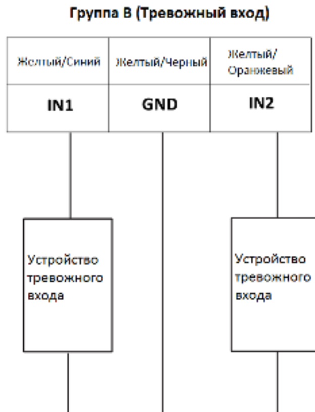
Рисунок 4-7 Подключение тревожного входа
