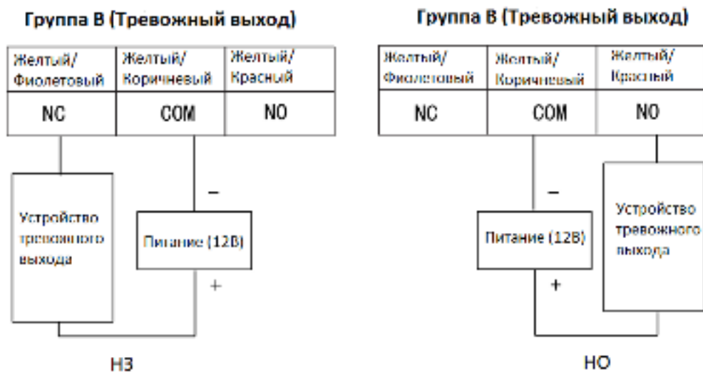
Рисунок 4-8 Установка внешнего тревожного устройства
