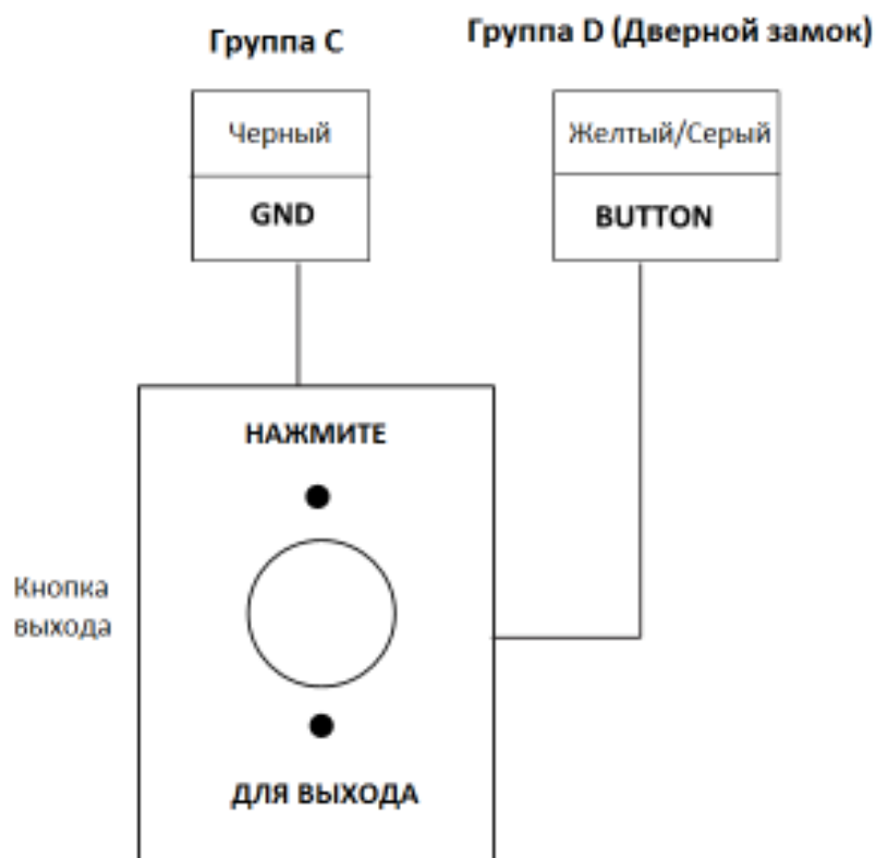
Рисунок 4-6 Установка кнопки выхода
