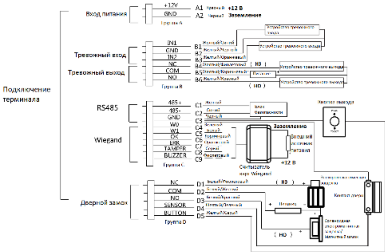
Рисунок 4-1 Подключение внешних устройств
