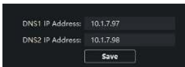
Рисунок 2-19. Настройки DNS
