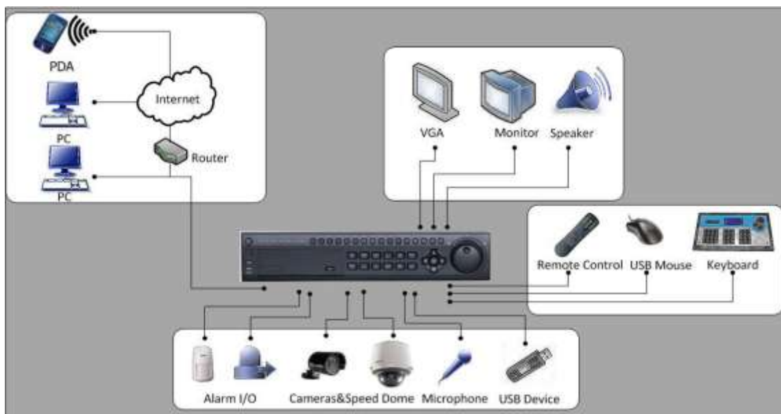
Рис. 2. Диаграмма подключений цифрового регистратора
