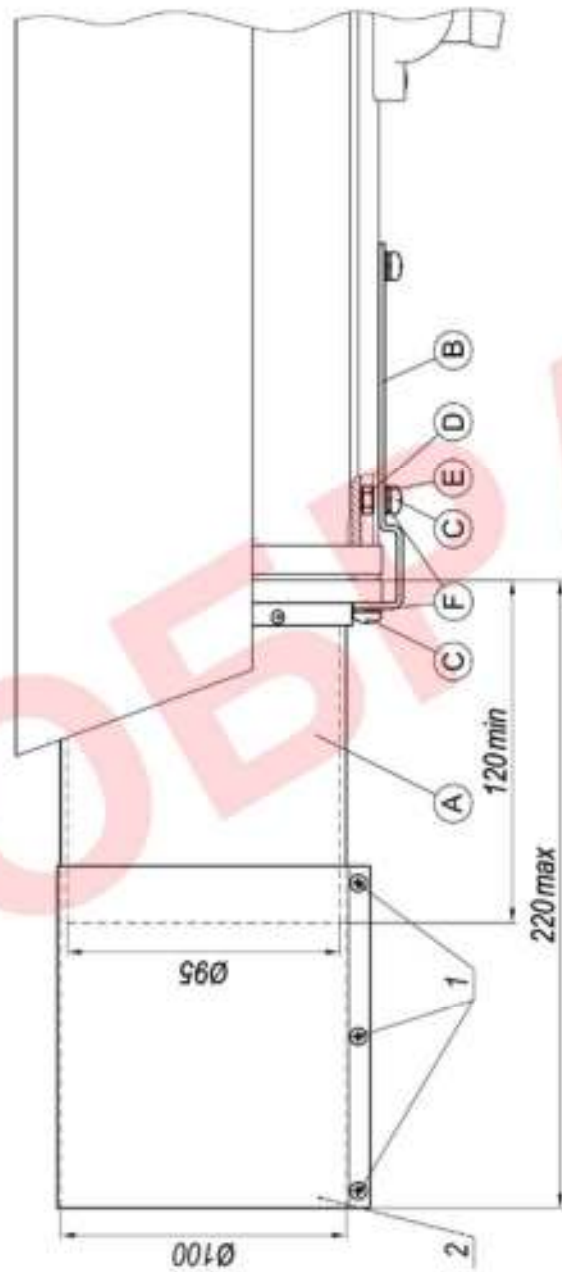
Рис.1 Установка бленды защитной на видеокамеры в термокожухах ТГБ-4Г Ex, ТГБ-4Р Ex
