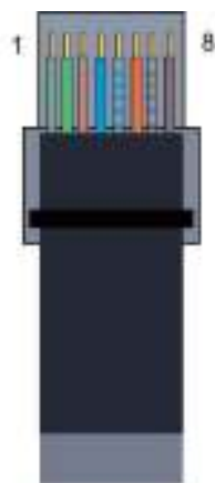
EIA/TIA 568A
