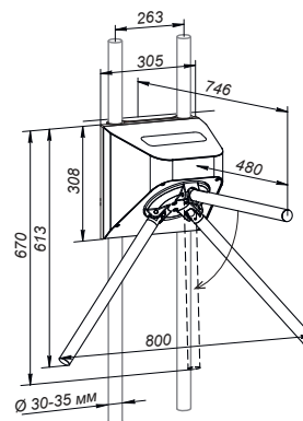
Габаритные размеры турникета TTR-10AT
