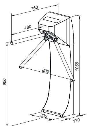
Габаритные размеры турникета TTR-10AB
