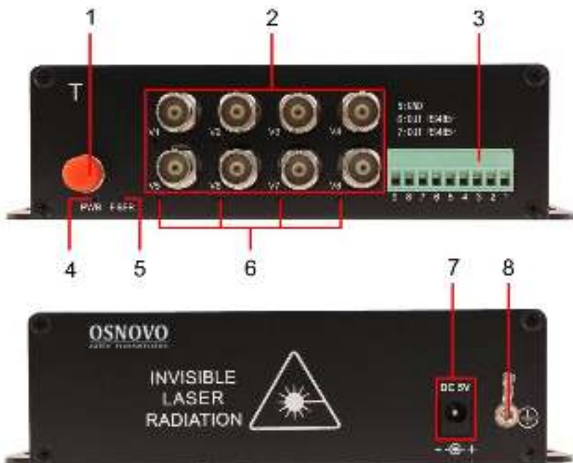
Рис.9 Разъемы подключения и индикаторы передатчика ТА-Н82-15F / приемника РА-Н82-15F
