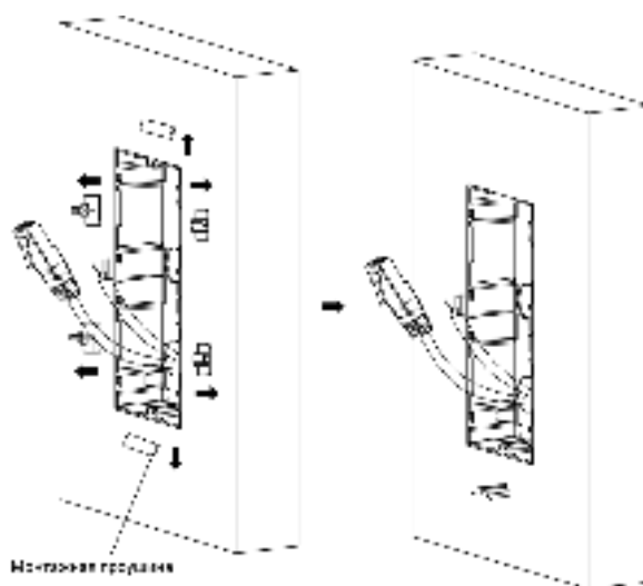
Рисунок 3-26 Извлечение монтажных проушин
