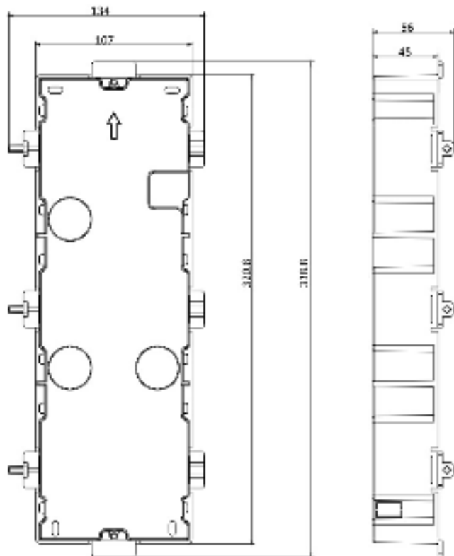
Рисунок 3-37 Монтажная коробка
