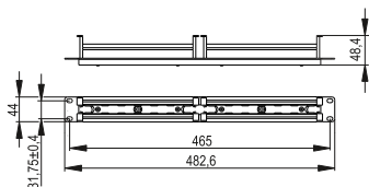
Рисунок 1 – CP100-1U110 (кросс-панель)
