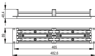
Рисунок 2 – CP200-2U110 (кросс-панель)
