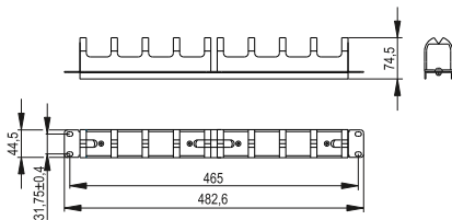
Рисунок 7 – CO35-1M110R (органайзер)
