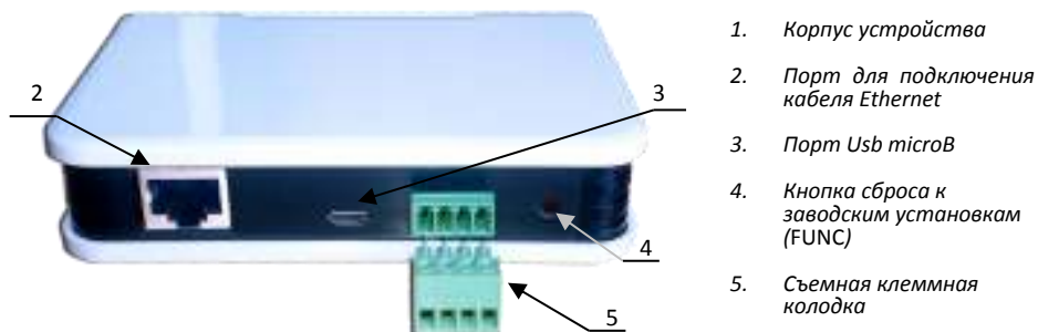
Рис. 1б. Внешний вид Gate-Hub Ethernet
