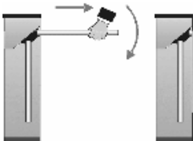
Рисунок 13. Использование преграждающих планок Антипаника
