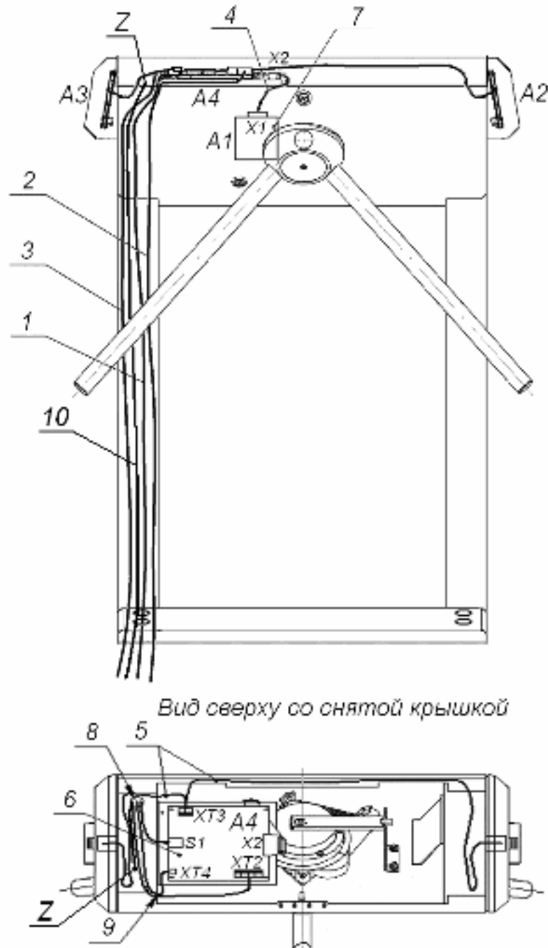
Рисунок 11. Схема прокладки кабелей в стойке ЭП
