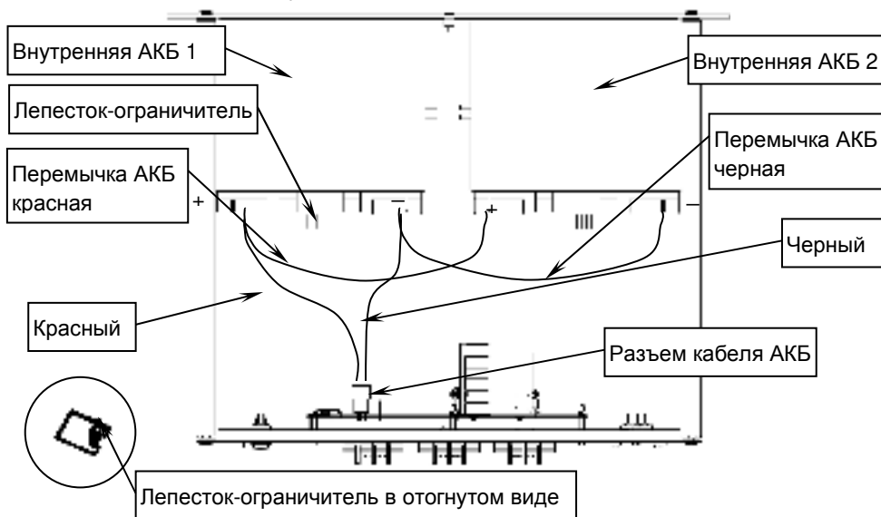
Рисунок 4 – Вид изделия со снятой крышкой и установленными АКБ
