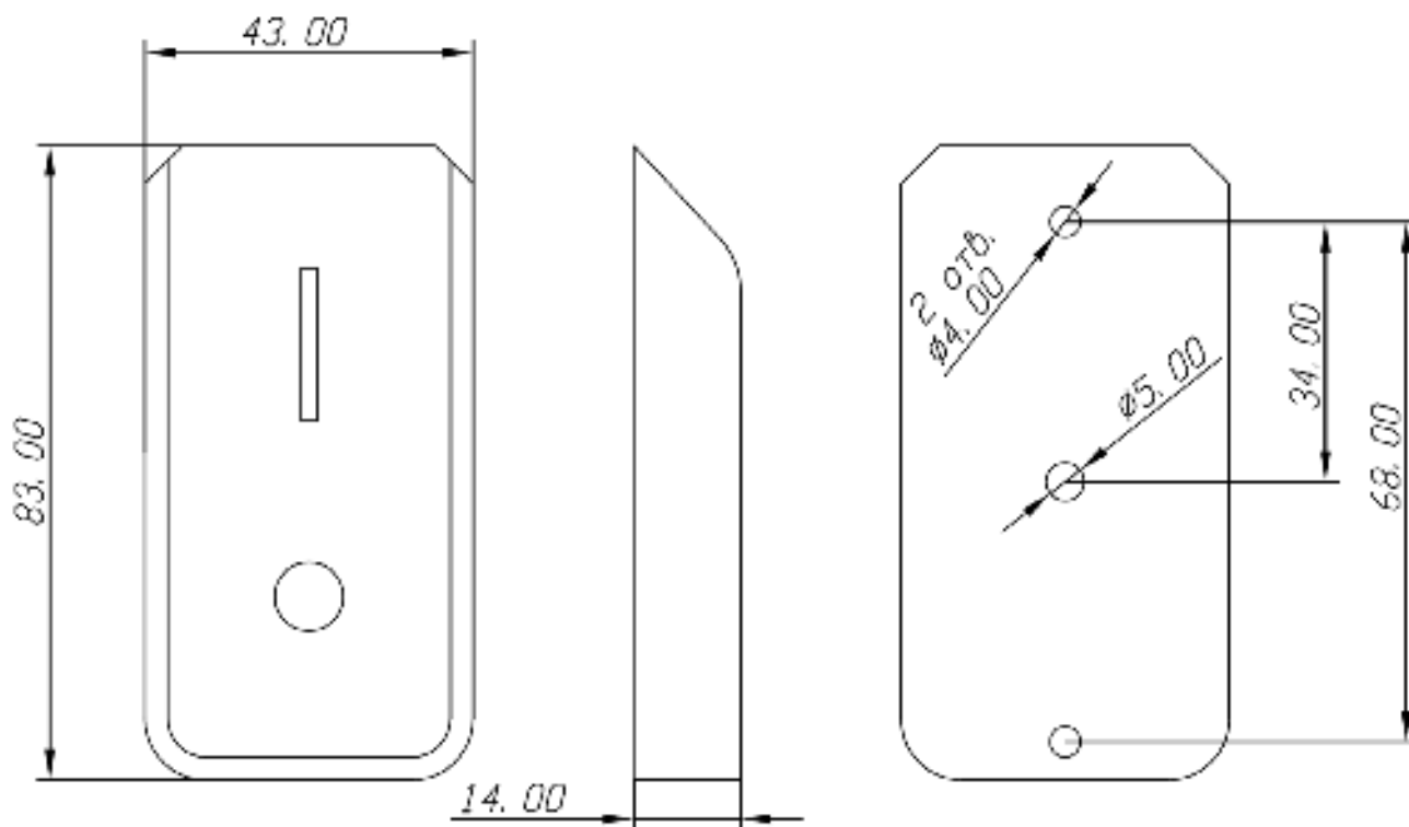
Рисунок 1. Внешний вид и габаритные размеры считывателя
