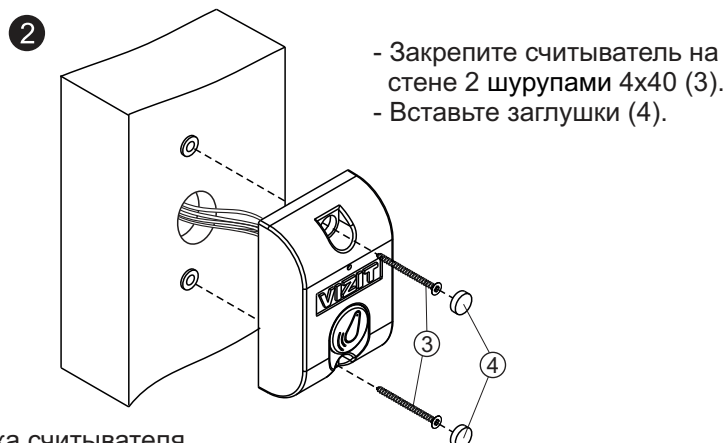
Рисунок 1 - Установка считывателя
