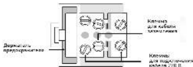
Рисунок 8. Клеммная колодка для кабеля питания
