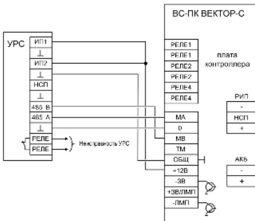
Рис.А3. Схема подключения устройства регистрации событий к прибору и РИП к УРС
