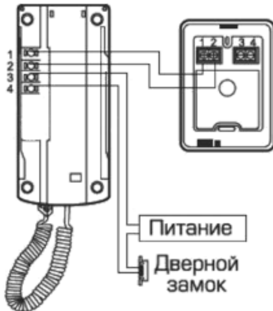
Схема подключения DP-2S
