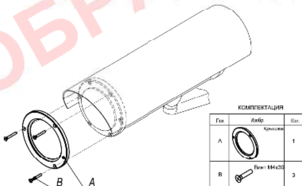
Рис.1 Установка HC-4 на термокожухи серии ТГБ-4Г(Р) Ex
