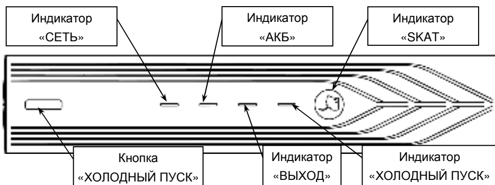
Рисунок 1 — Общий вид передней панели источника
