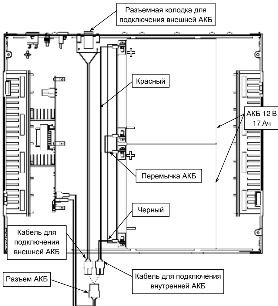
Рисунок 4 – Схема размещения и подключения внутренней АКБ, состоящей из двух аккумуляторных батарей 17Ач 12В, соединенных последовательно
