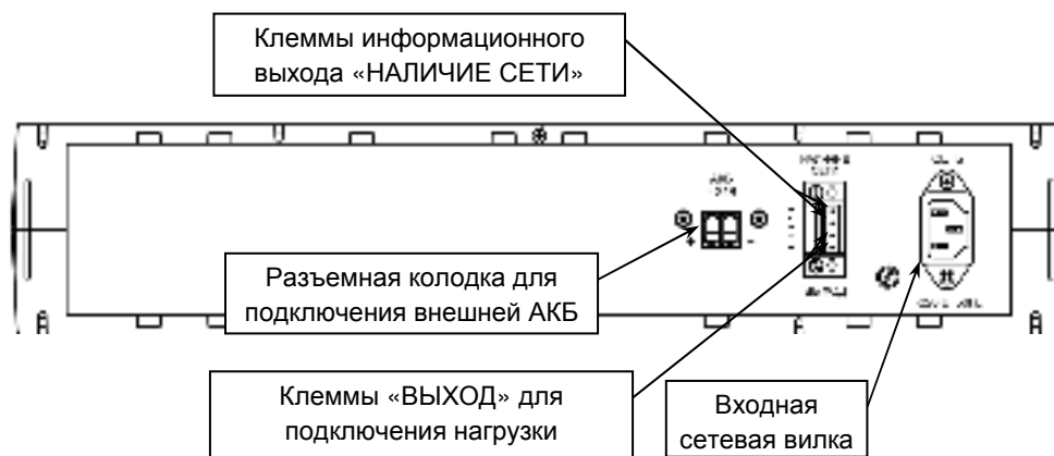
Рисунок 2 — Общий вид задней панели источника
