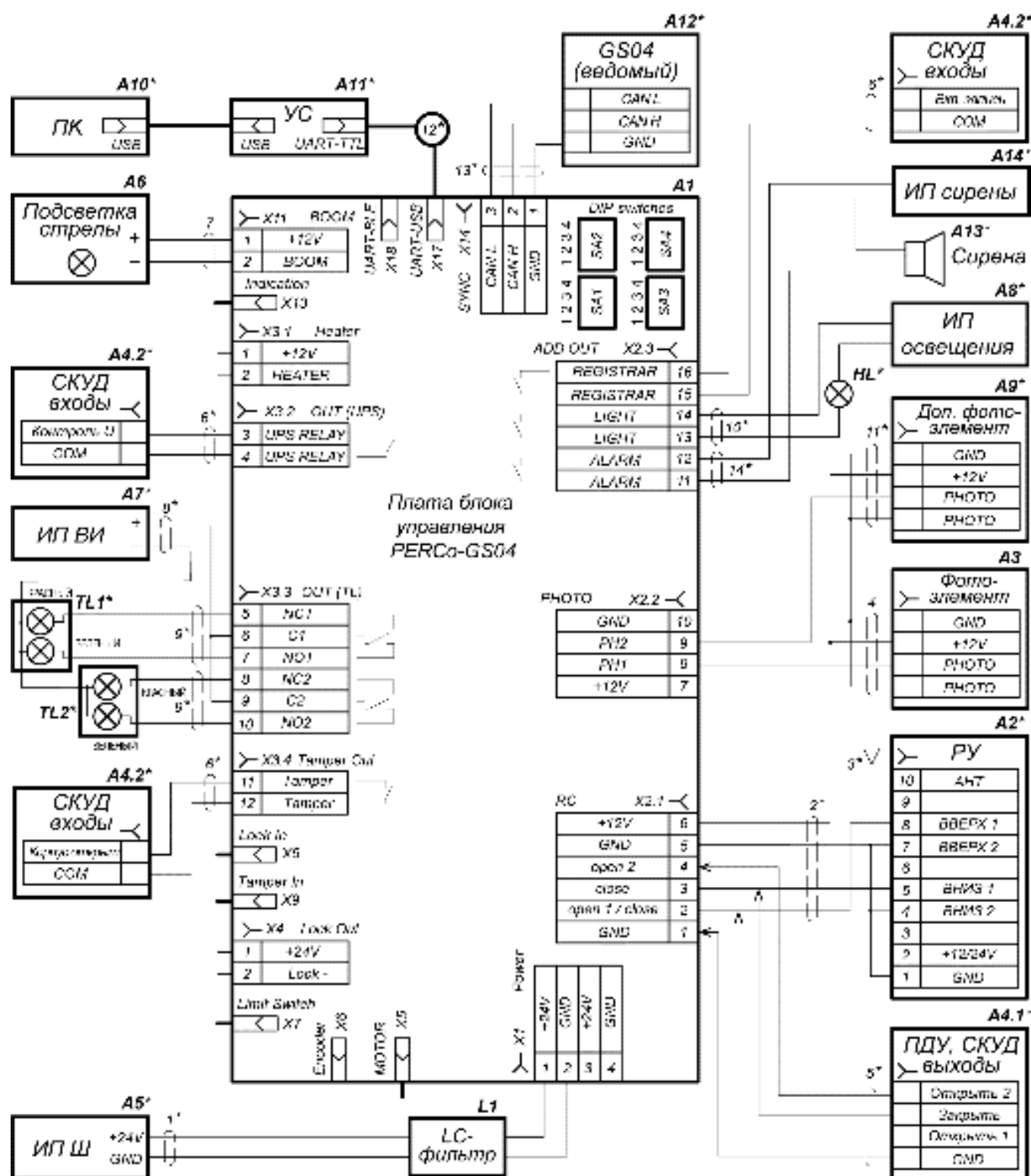
Рисунок 24. Схема подключения шлагбаума и доп. оборудования (перечень элементов см. в табл. 4)
