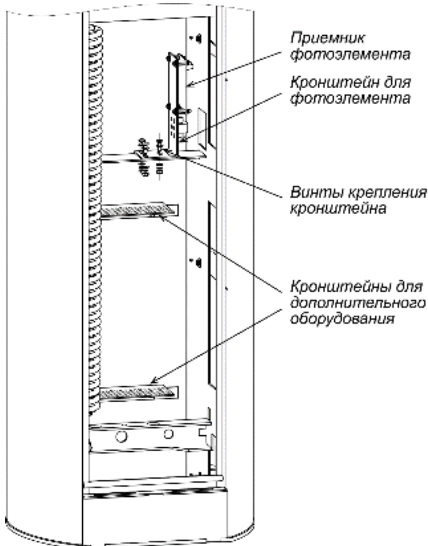
Рисунок 21. Установка фотоэлемента безопасности и доп. оборудования
