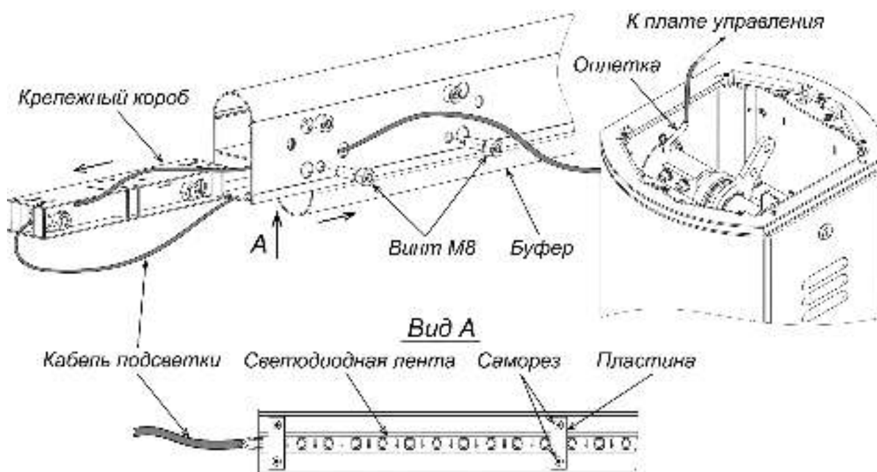
Рисунок 19. Монтаж подсветки стрелы PERCo-GBS1
