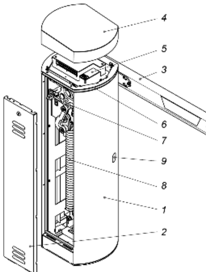
Рисунок 2. Устройство шламбаума
