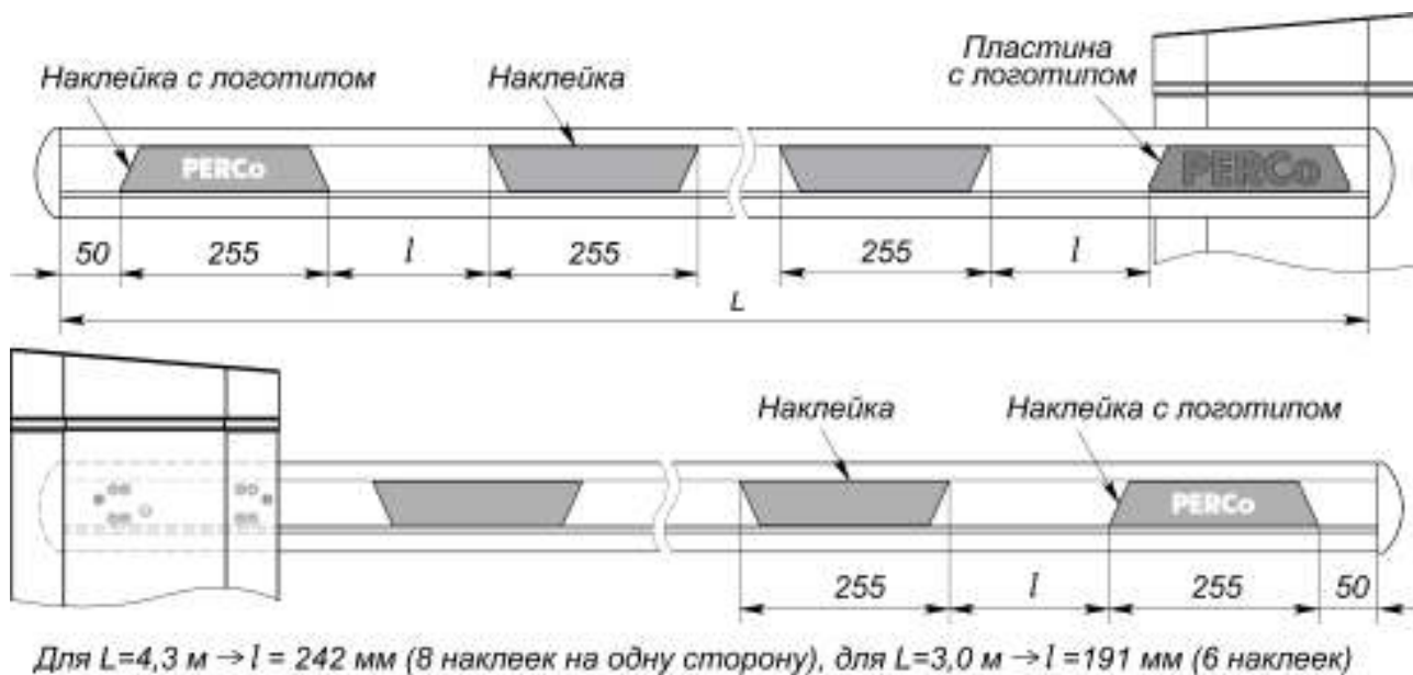
Рисунок 12. Наклеивание световозвращающих элементов на стрелу PERCo-GBO
