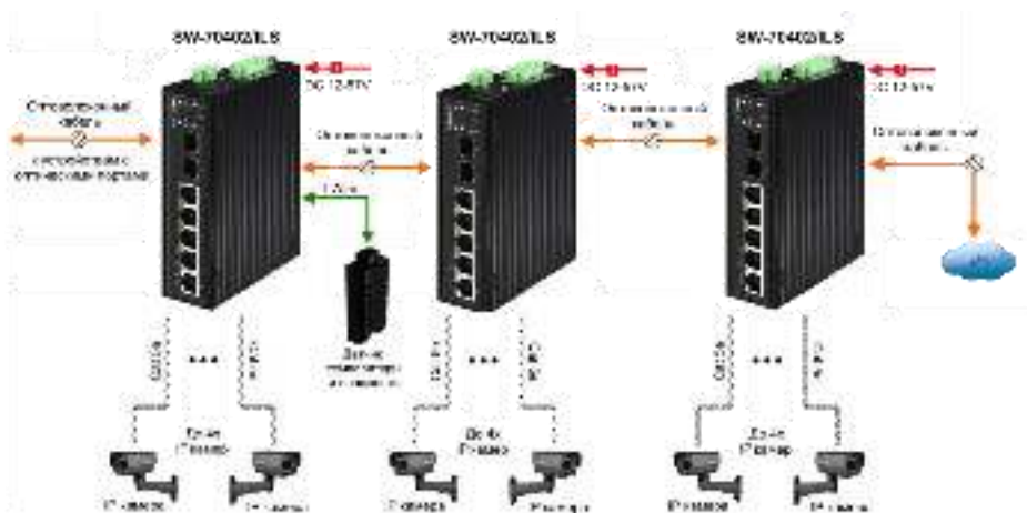
Рис.11 Схема подключения коммутатора каскадом, на примере SW-70402/ILS
