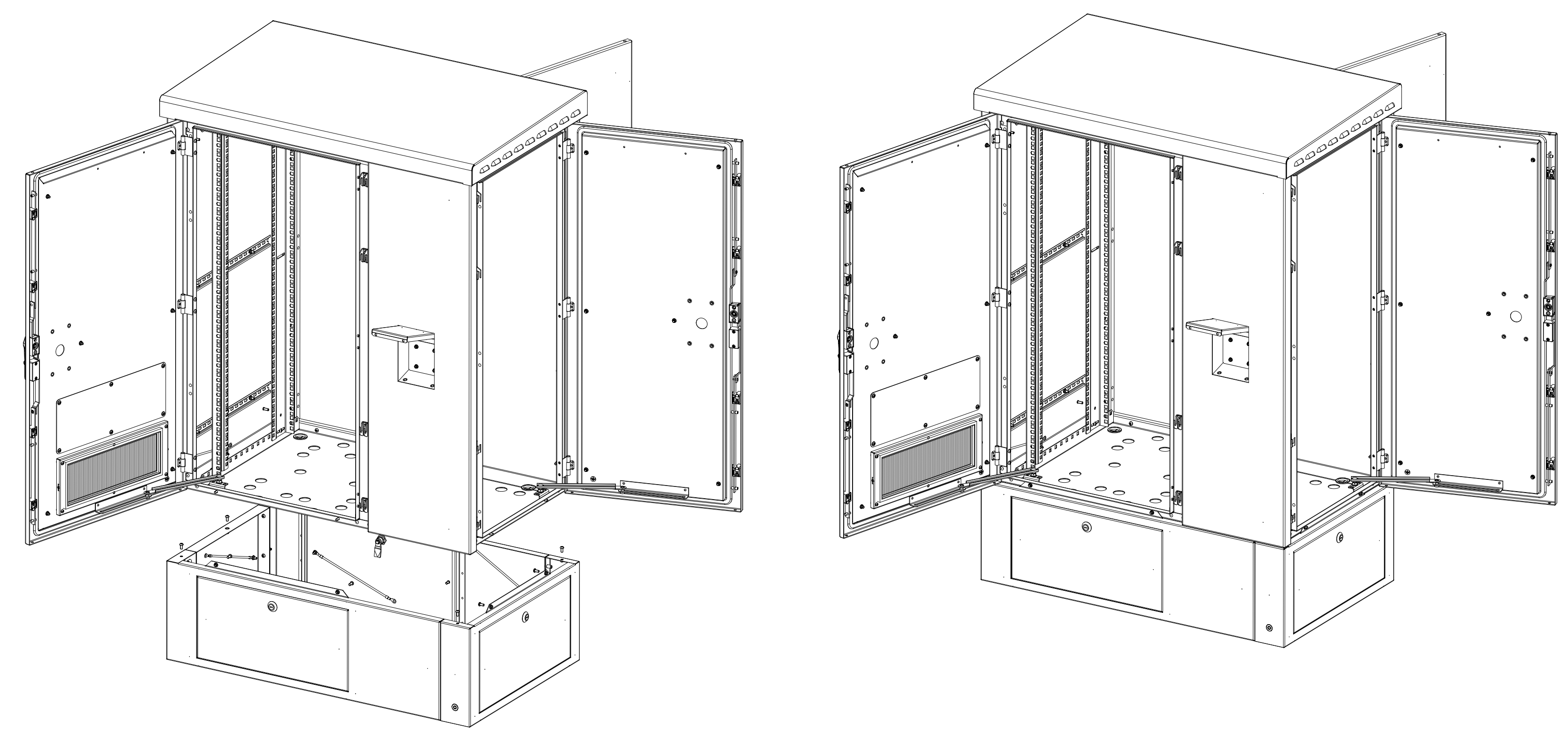
Установка цоколя ОС-ШТВ-2-300.x на базовый цоколь 100мм: 7 винтов М6х12 + 6 заек М6
