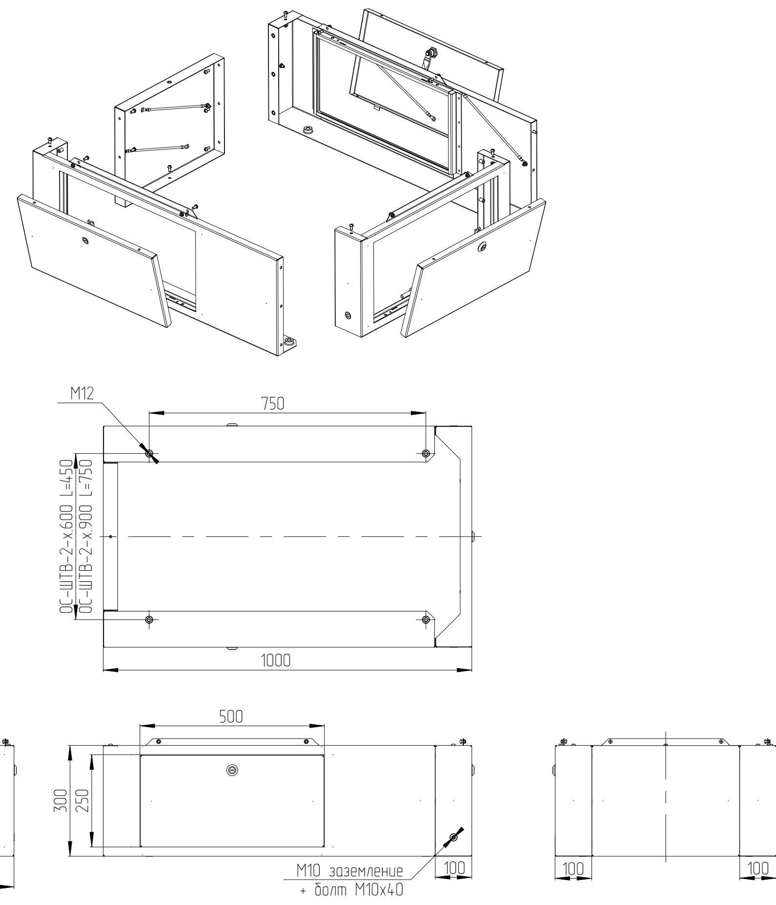
Цоколь ОС-ШТВ-2-300.600 и Цоколь ОС-ШТВ-2-300.900
