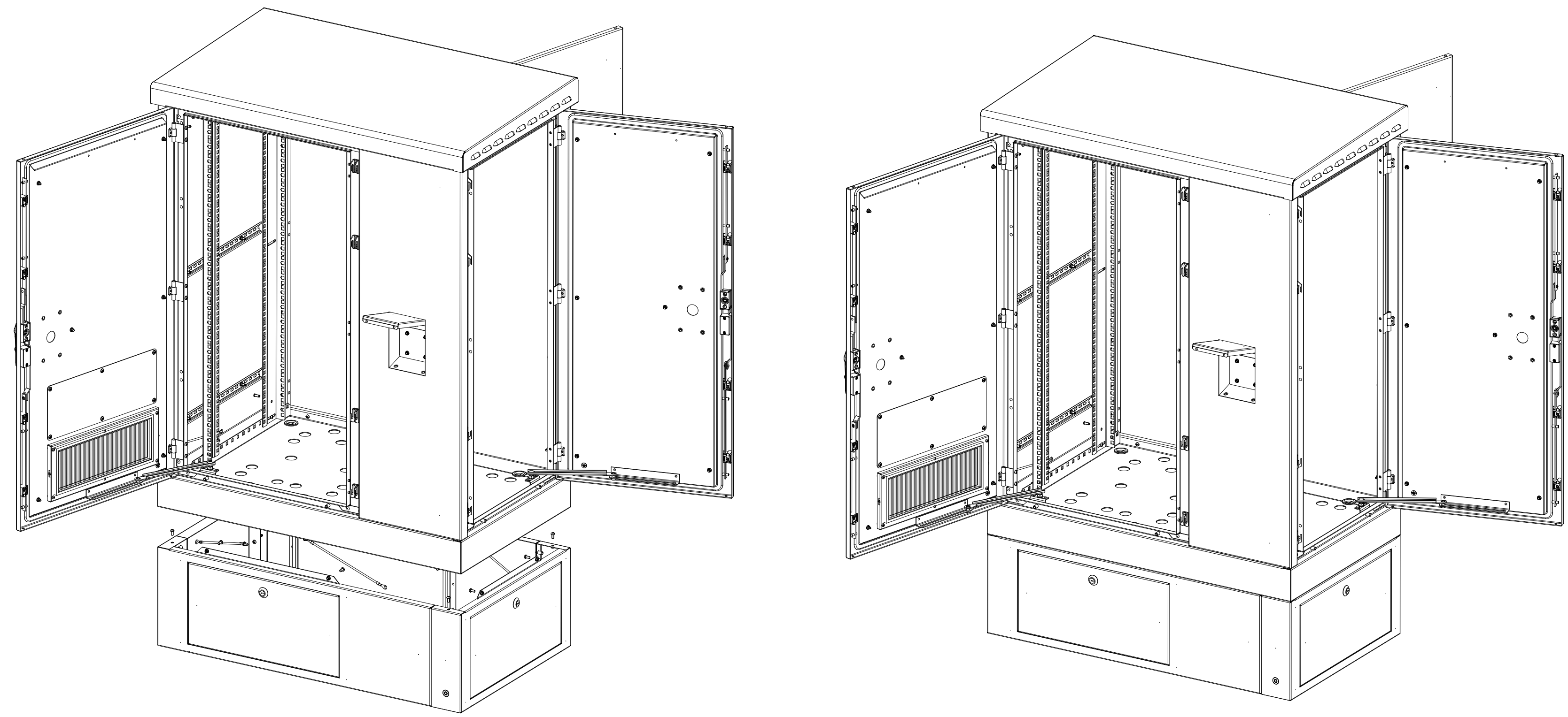
Установка цоколя ОС-ШТВ-2-300.x на базовый цоколь 100мм: 11 винтов М6х12 + 6 заек М6
