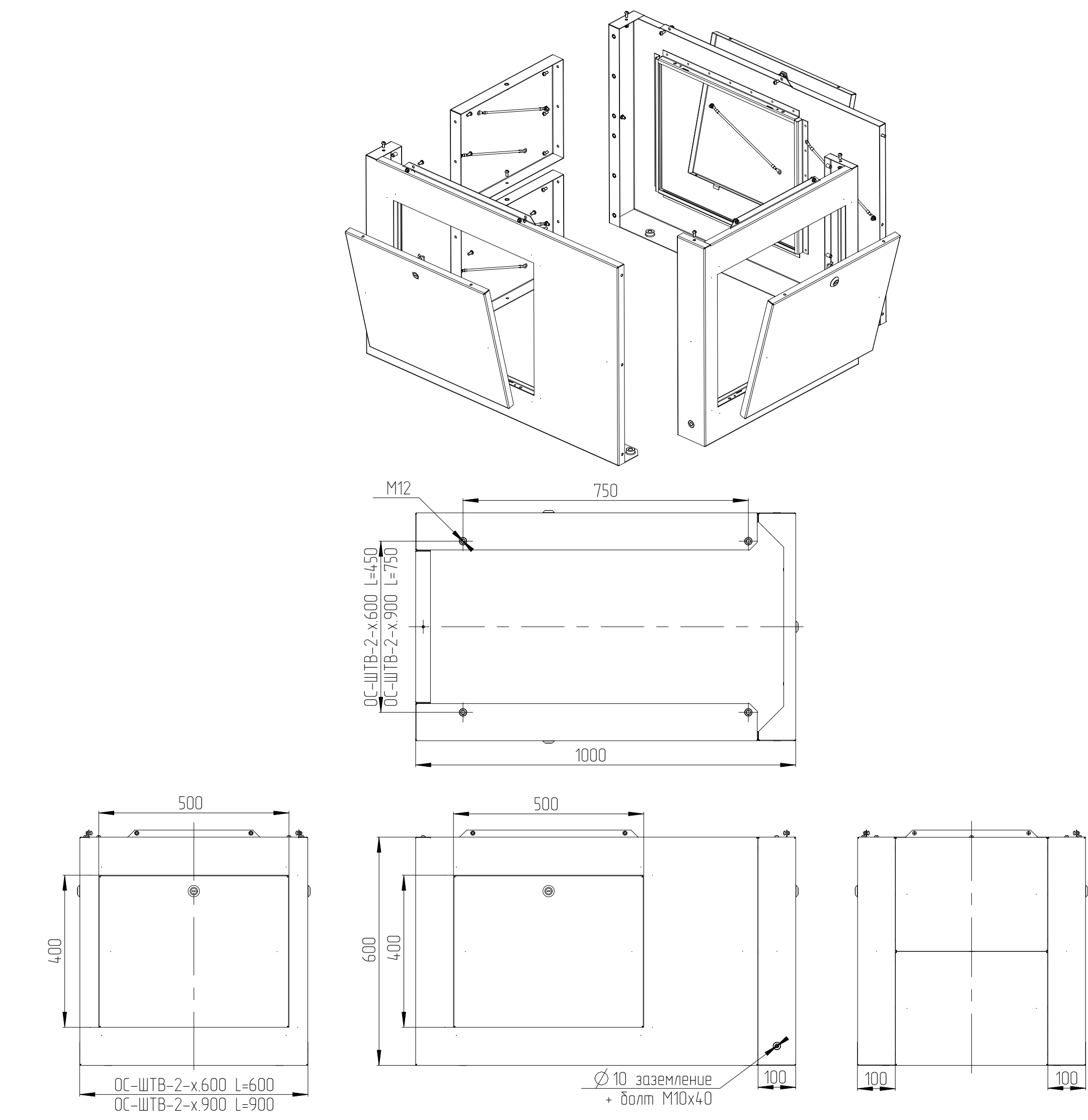
Цоколь ОС-ШТВ-2-600.600 и Цоколь ОС-ШТВ-2-600.900
