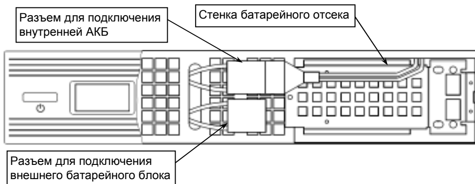
Рисунок 5 – Подключение внутренних батарей
