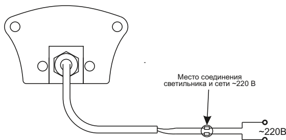
Рисунок 2 — Схема подключения изделия
