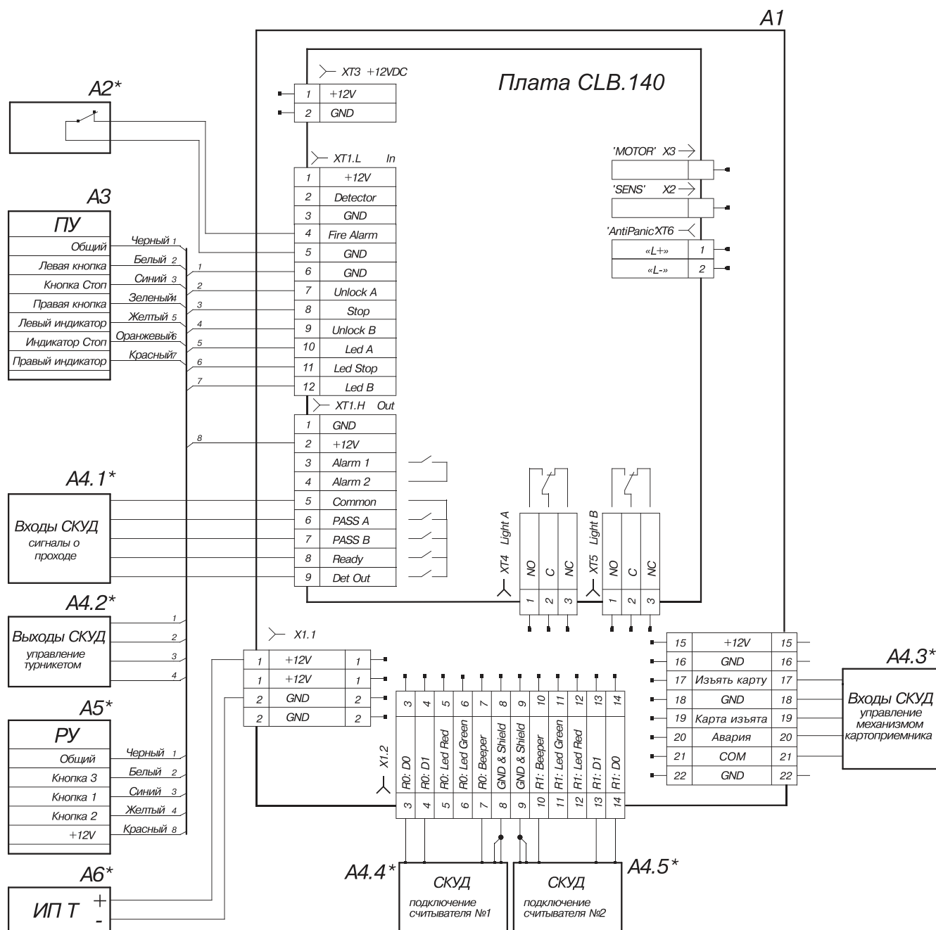
Схема соединений турникета PERCo-TBC01.9A и дополнительного оборудования
