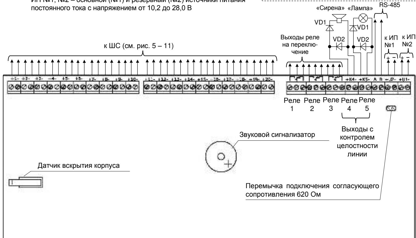
Рисунок 4. Схема внешних соединений прибора «Сигнал-20М»
