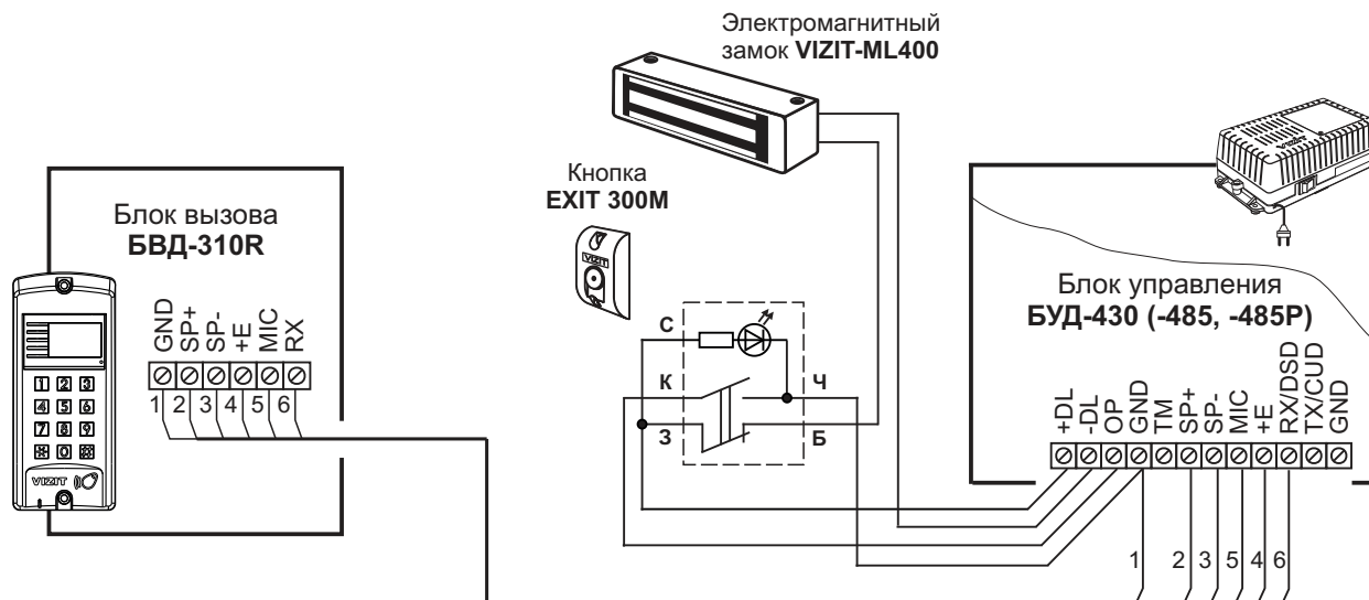
Рисунок 8 - Схема соединений блока вызова БД-310R с блоком управления БУД-430 (-485, -485P) , электромагнитным замком VIZIT-ML400 и кнопкой “EXIT 300M”
