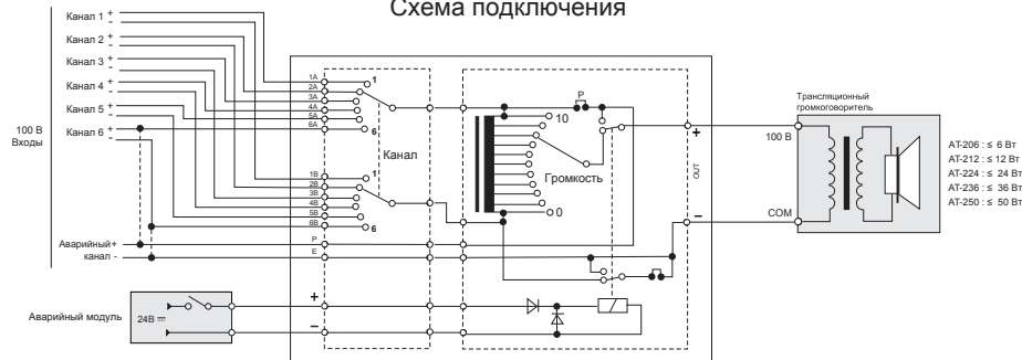
Схема подключения
