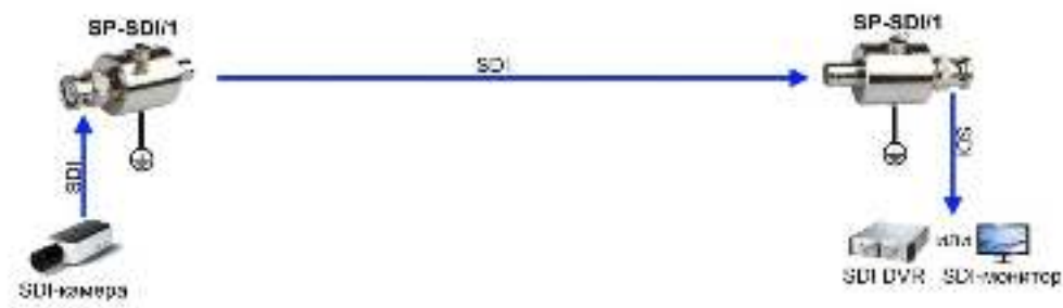
Рис. 5 Схема подключения SP-SDI/1.
