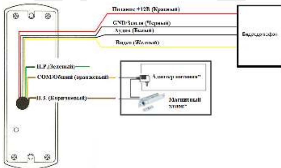
Рис. 2. Схема подключения
