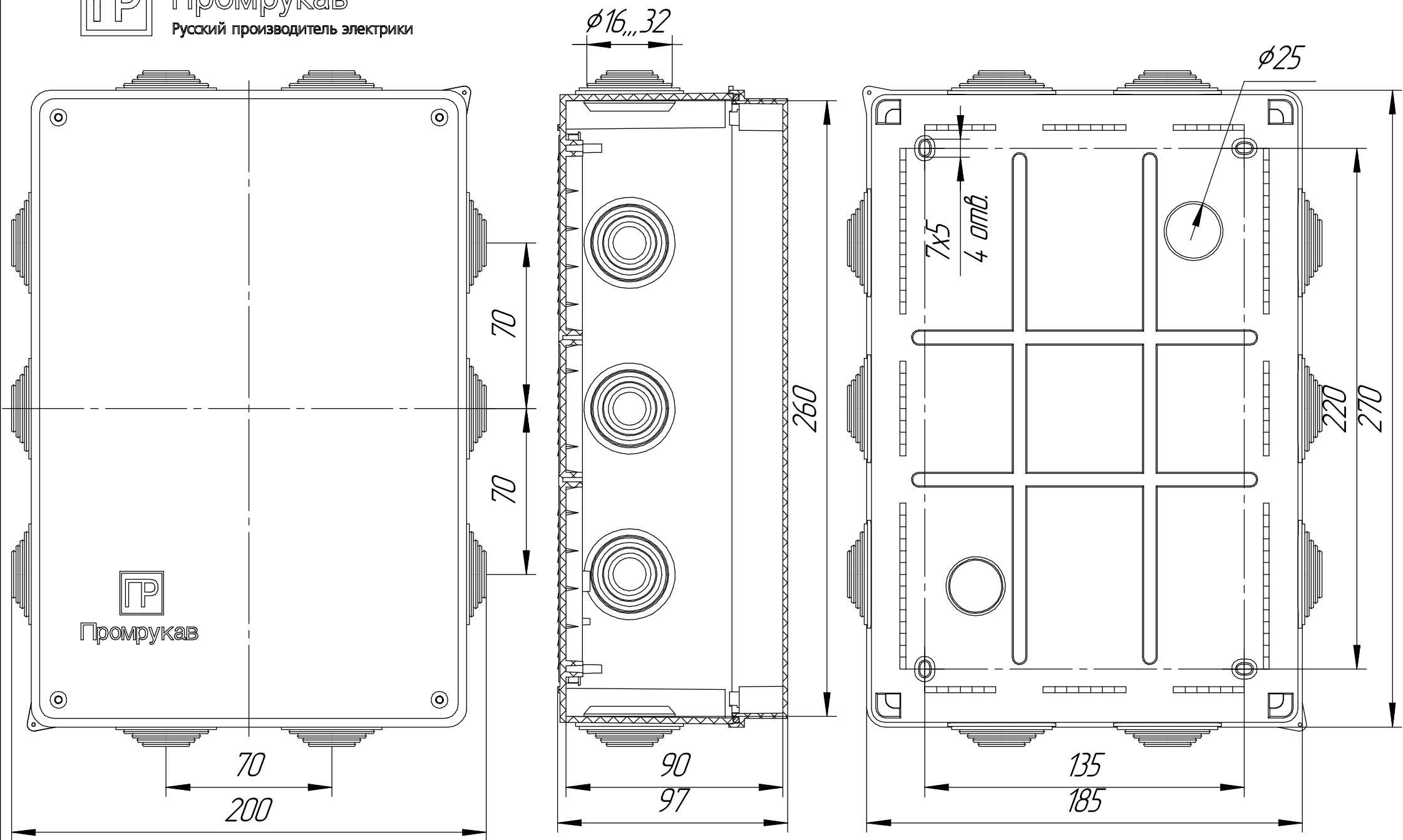
Коробка распределительная 40-0330 для о/п безгалогенная (HF) 260x175x90
