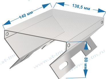
Рис.1 Габаритные размеры
